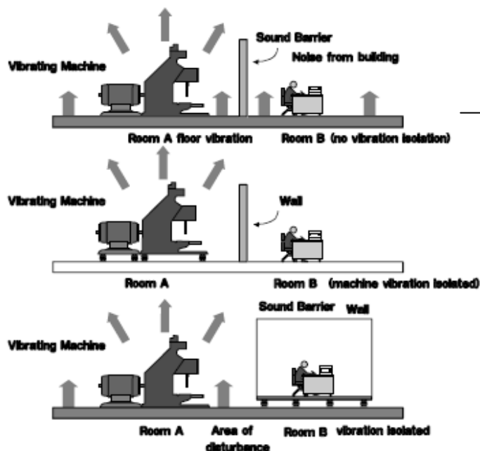
شکل شماره 3- نمایی از ایزولاسیون ارتعاش دستگاه به اشکال مختلف
