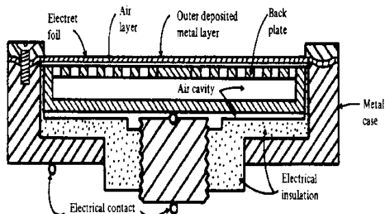
شکل شماره 3- نمایی از ساختار میکروفن الکتره
