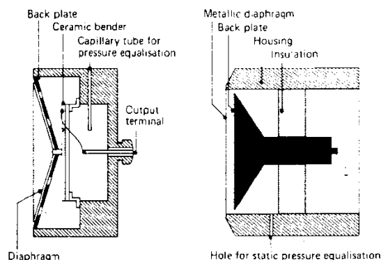
شکل شماره 2- نمایی از ساختار میکروفن کریستالی
