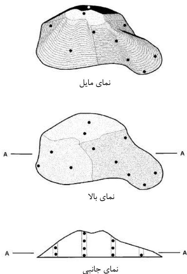
شکل ۳- راهبرد نمونه‌برداری توده پسماند- نمونه‌برداری تصادفی لایه‌ای
