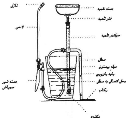
تصویر ۲۳: اجزای تشکیل دهنده یک پمپ رکابی
