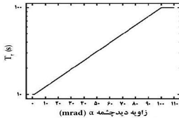
شکل ۹- بستگی T_v به زاویه دید چشمه
