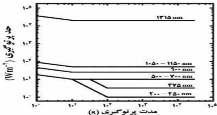
شکل ۱۲- نمودار حدود پرتوگیری چشم با لیزرهای پیوسته به عنوان منابع نور نقطه ای در محدوده طول موج های ۴۰۰ الی ۱۴۰۰ نانومت
